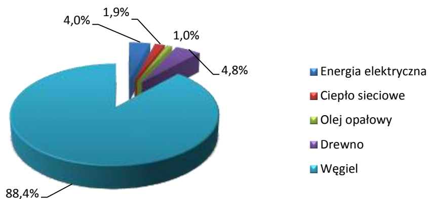
Rysunek 35 Struktura zużycia nośników energii w sektorze mieszkaniowym na terenie Gminy Bierawa w roku bazowym 2013 241
