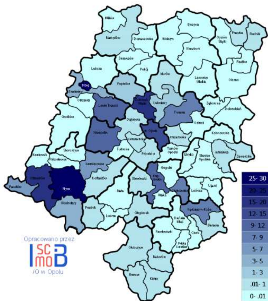
Rysunek 21 Potencjał wód powierzchniowych województwa opolskiego [GWh/rok] 181
